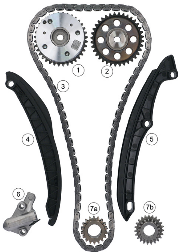
Figuur 1: 559 1808 40 / 559 1808 41 – onderdelen distributieketting-KIT
