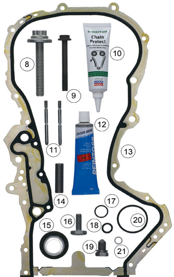
Figuur 2: toebehoren distributieketting-KIT 559 1808 40 / 559 1808 41
